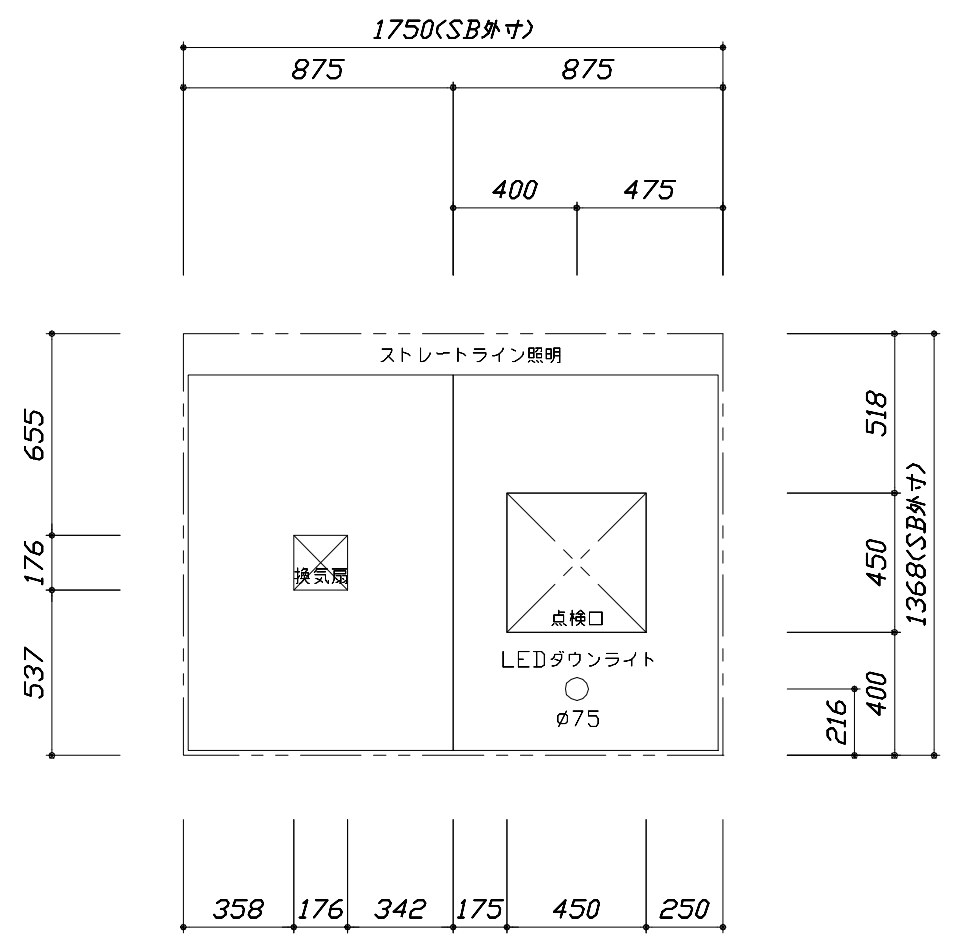
<天井伏図>
